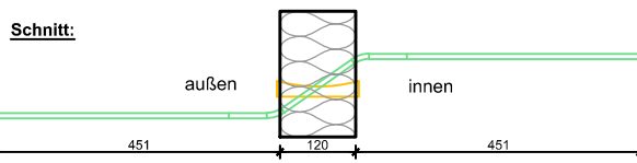
Schöck Isokorb Typ QXT60
