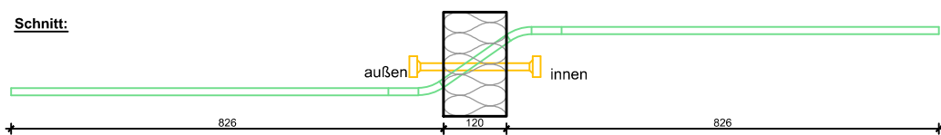
Schöck Isokorb Typ QPXT60 - QPXT100
