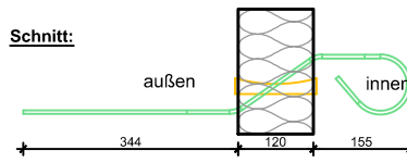
Schöck Isokorb Typ QXT10 - QXT40
