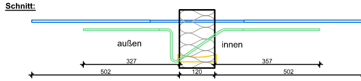
Schöck Isokorb Typ K(F)XT15-V6-V8 - K(F)XT50-V6-V8
