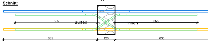
Schöck Isokorb Typ DXT30 - DXT90
