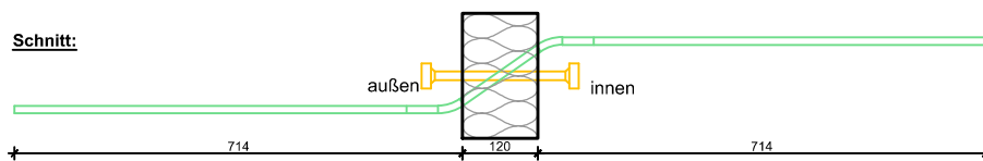
Schöck Isokorb Typ QPXT40 + QPXT50
