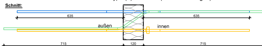
Schöck Isokorb Typ E(F)XT50-V12 (=max. Stablängen)
