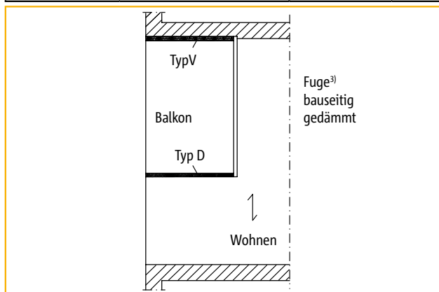
Abbildung 1: Decke einachsig gespannt
