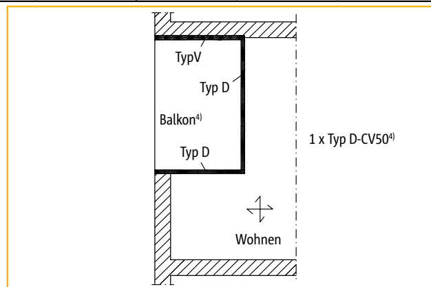
Abbildung 2: Decke kreuzweise gespannt, Einspannungswirkung Schöck Isokorb® ist jedoch nur einachsig vorhanden
