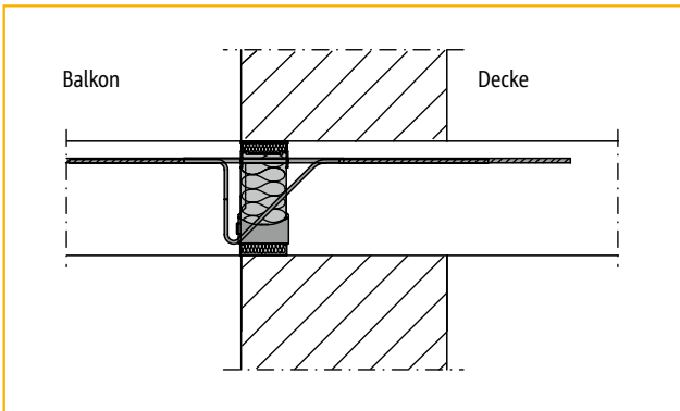
Abbildung 5: Einschaliges Mauerwerk bei deckengleichem Balkon
