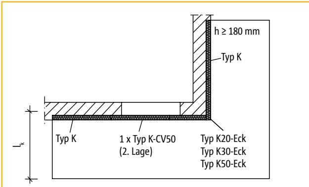
Abbildung 3: Balkon bei Außenecken
