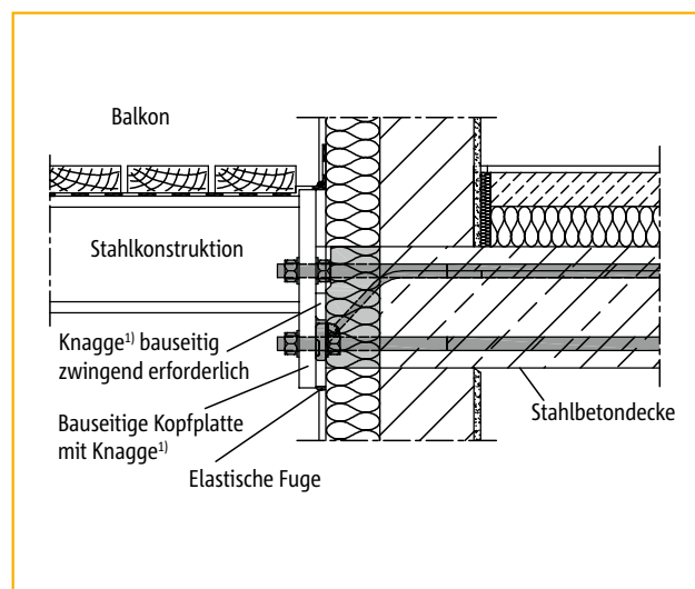
höhenversetzter Anschluss für barrierefreie Übergänge
