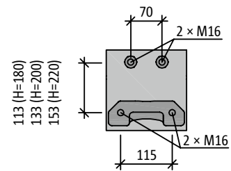
Vorderansicht: Schöck Isokorb® Typ KS 14 VV
