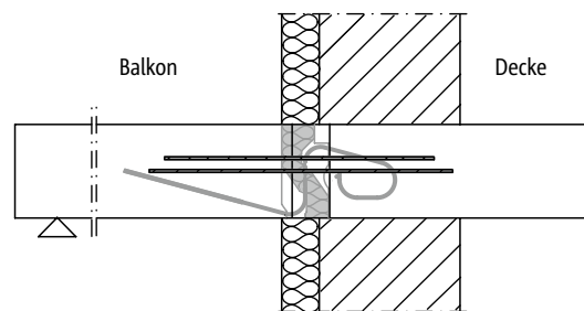
Abbildung 6: Mauerwerk mit Außendämmung bei deckengleichem Balkon + Typ V + Typ HPC-Modul
