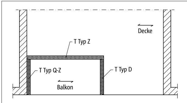
Abb. 278: Schöck Isokorb® T Typ D, QZ, Z: Decke einachsig gespannt
