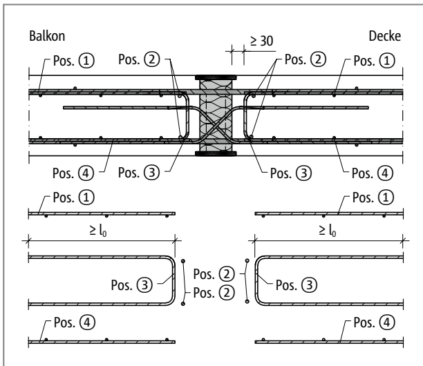
Abb. 290: Schöck Isokorb® T Typ D: Bauseitige Bewehrung
