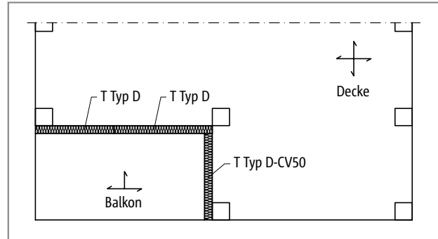
Abb. 279: Schöck Isokorb® T Typ D: Einsatz in Flachdecken
