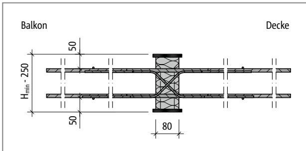
Abb. 285: Schöck Isokorb® T Typ D bei CV50: Produktschnitt
