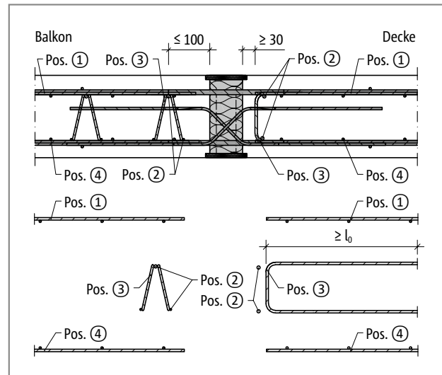
Abb. 291: Schöck Isokorb® T Typ D: Bauseitige Bewehrung mit Gitterträger
