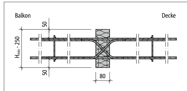
Abb. 289: Schöck Isokorb® T Typ D bei R0-CV50: Produktschnitt
