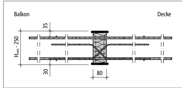
Abb. 284: Schöck Isokorb® T Typ D bei CV35: Produktschnitt
