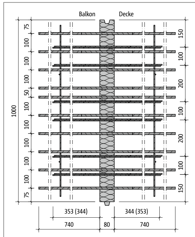
Abb. 287: Schöck Isokorb® T Typ D-MM4-VV1: Grundriss
