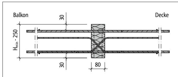
Abb. 288: Schöck Isokorb® T Typ D bei R0-CV30: Produktschnitt
