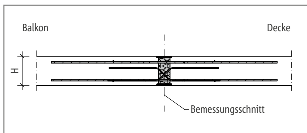
Abb. 282: Schöck Isokorb® T Typ D: Statisches System
