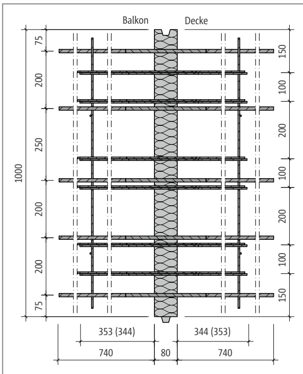
Abb. 286: Schöck Isokorb® T Typ D-MM2-VV1: Grundriss
