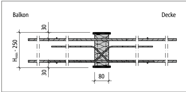
Abb. 283: Schöck Isokorb® T Typ D bei CV30: Produktschnitt
