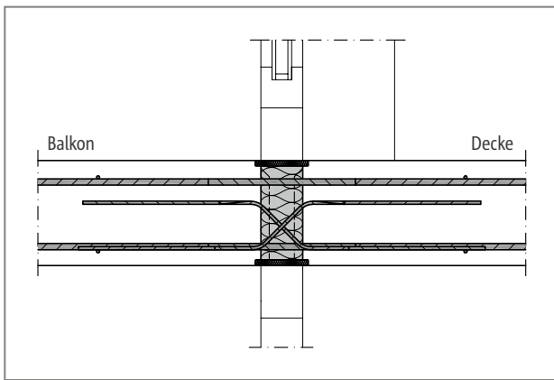
Abb. 280: Schöck Isokorb® T Typ D: Einbauschnitt; einachsig gespannte Decke
