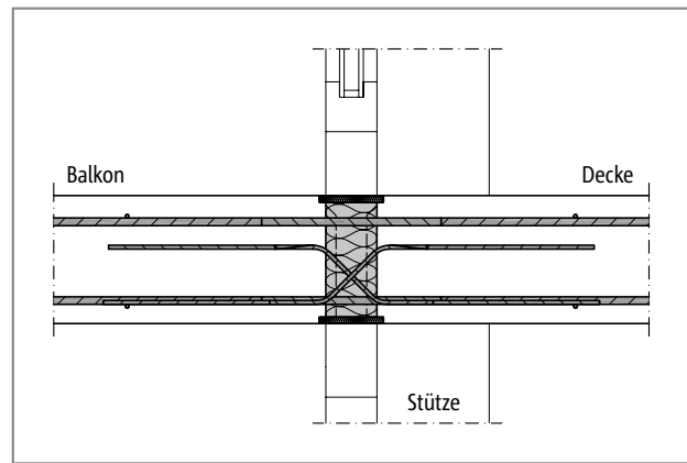
Abb. 281: Schöck Isokorb® T Typ D: Einbauschnitt; Flachdecke
