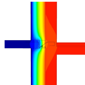
Isothermenbild des XT Typ K-BH-M2-V1
