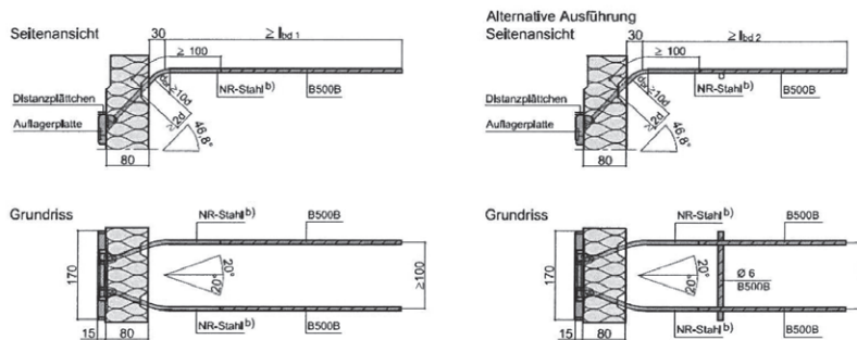
Abb. 14a bis 14d: Querkraftstäbe 2 Ø 8 Inkl. Auflagerplatte
