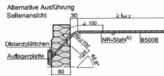
Abb. 8: Drucklager 2 Ø 14
