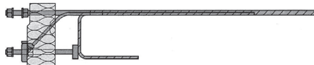
Abb.1 Schöck Isokorb Typ KS14 V8 und KS14 V10
