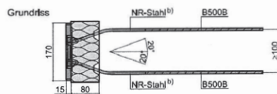
Abb. 9a bis 9d: Querkräftstäbe 2 Ø d inkl. Auflagerplatte
