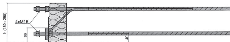
Abb. 38 Seitenansicht: Schöck Isokorb Typ KS14 VV
