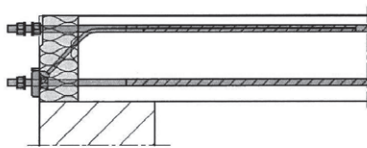
Abb. 46 Seitenansicht: Schöck Isokorb Typ KS14 VV
