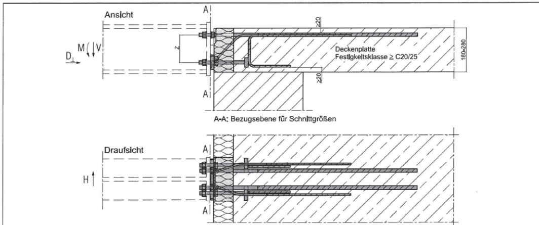
Abb. 27 und 28: Schöck Isokorb Typ KS14 V8 und KS14 V10, Schnittgrößendefinition
