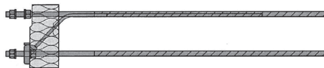
Abb.2 Schöck Isokorb Typ KS14 VV
