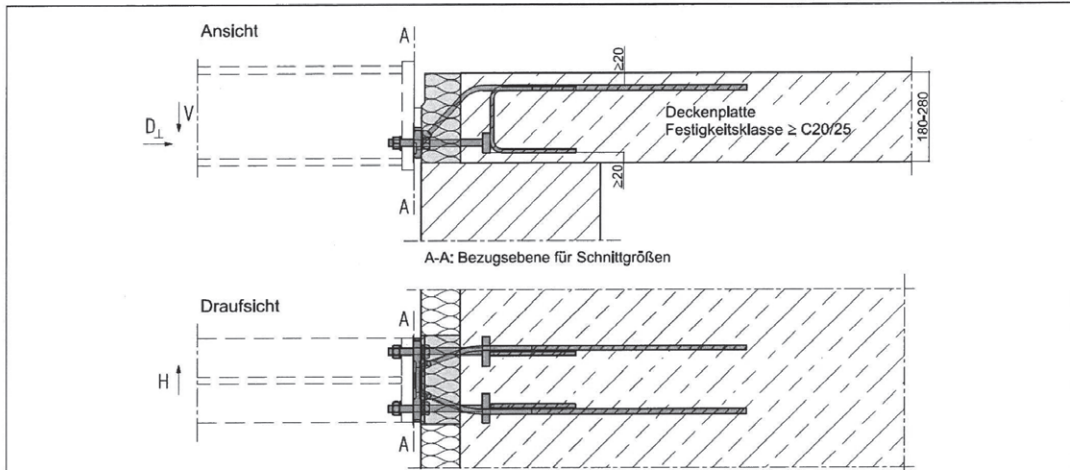
Abb. 33 und 34: Schöck Isokorb Typ QS10 und QS12, Schnittgrößendefinition
