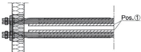
Abb. 47 Draufsicht: Schöck Isokorb Typ KS14 VV
