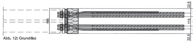
Abb. 12: Grundriss
