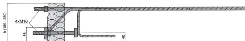
Abb. 37 Seitenansicht: Schöck Isokorb Typ KS14 V8 und KS14 V10
