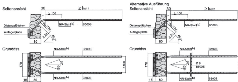
Abb. 20a bis 20d: Querkraftstäbe 2 Ø d inkl. Auflagerplatte
