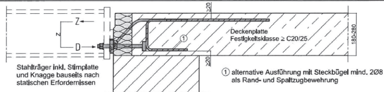
Abb. 22: Schöck Isokorb Typ QS10 und QS12
