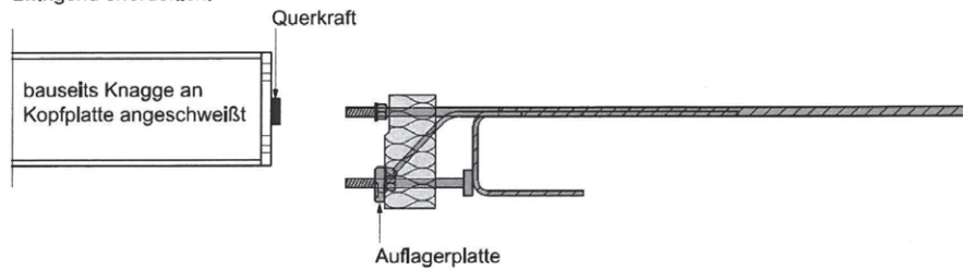
Abb. 36 Querkraftübertragung durch Knagge
