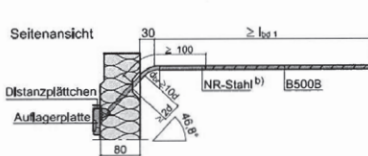
Abb. 7: Zugstäbe 2 Ø 14
