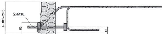
Abb. 42 Seitenansicht: Schöck Isokorb Typ QS10 und QS12
