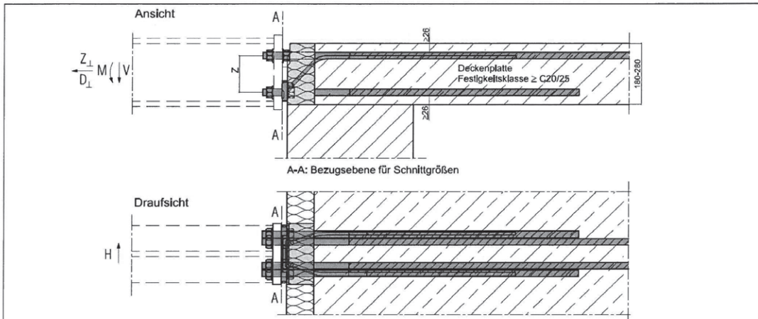
Abb. 31 und 32: Schöck Isokorb Typ KS20, Schnittgrößendefinition
