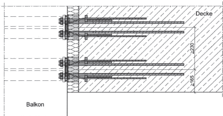
Abb. 35 Achs- und Randabstände
