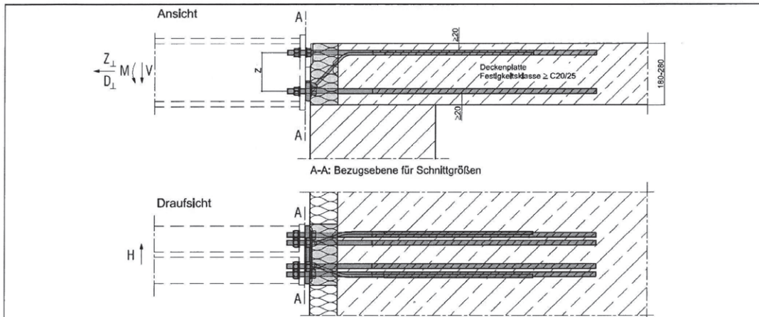
Abb. 29 und 30: Schöck Isokorb Typ KS14 VV, Schnittgrößendefinition
