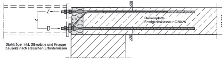
Abb. 11: Schöck Isokorb Typ KS14 VV
