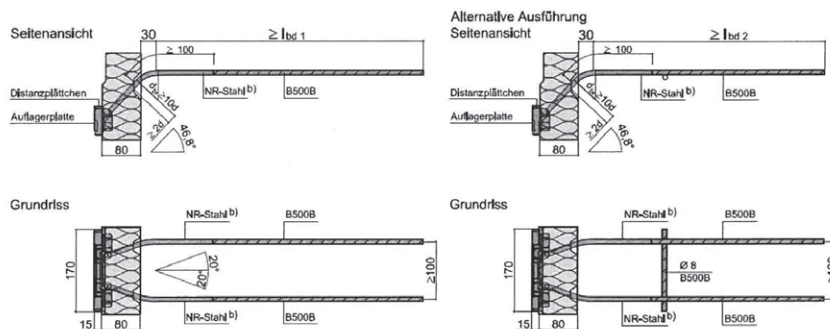
Abb. 25a bis 25d: Querkraftstäbe 2 Ø d inkl. Auflagerplatte
