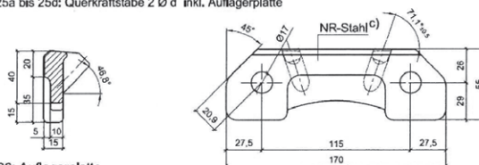
Abb. 26: Auflagerplatte
