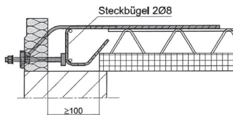
Abb. 49 Bauseitige Anschlussbewehrung für Schöck Isokorb Typ QS mit hochgebogenem Steckbügel
