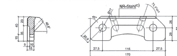
Abb. 15: Auflagerplatte
