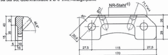
Abb. 10: Auflagerplatte
