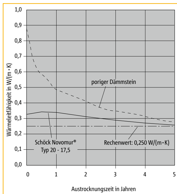
Abb. 8: Änderung der Wärmeleitfähigkeit während der Austrocknungsphase am Beispiel eines porigen Dämmsteins und Schöck Novomur® Typ 20-17,5
