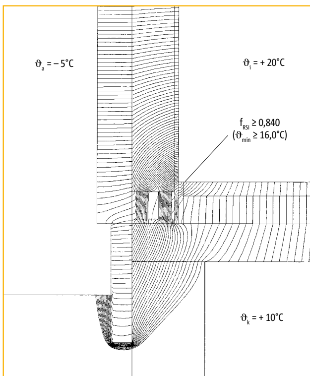
Wärmestromlinien, Temperaturfaktor und minimale Oberflächentemperatur bei Wärmedämmverbundsystem
