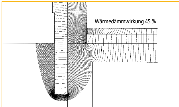
Abb. 2b: Wärmestromlinien bei konstruktiver Dämmmaßnahme
