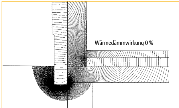
Abb. 1b: Wärmestromlinien bei ungedämmtem Gebäudesockel
