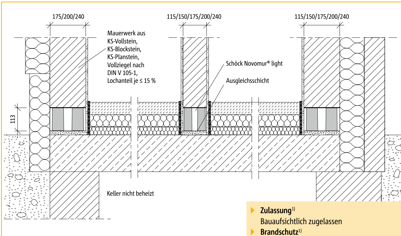
Einbauzustand Schöck Novomur® light bei Wärmedämmverbundsystem, Innenwand und zweischaliger Wand
