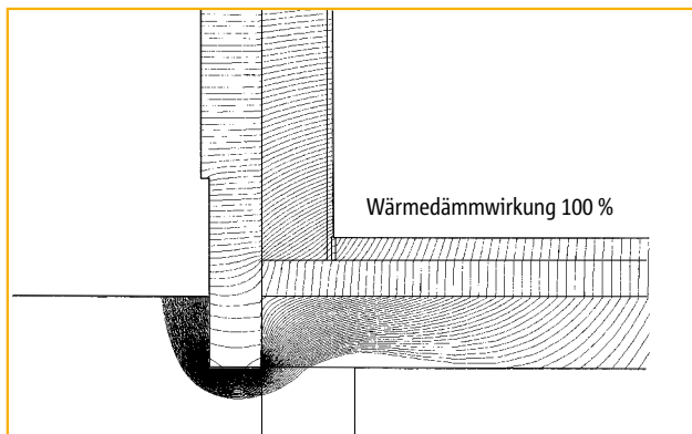
Abb. 4b: Wärmestromlinien bei theoretisch ideal gedämmtem Gebäudesockel
