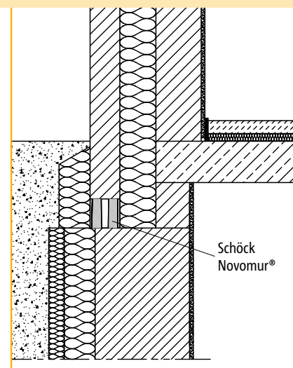
Einbauzustand Schöck Novomur® zweischalig (z.B. Klinkervormauerschale)
