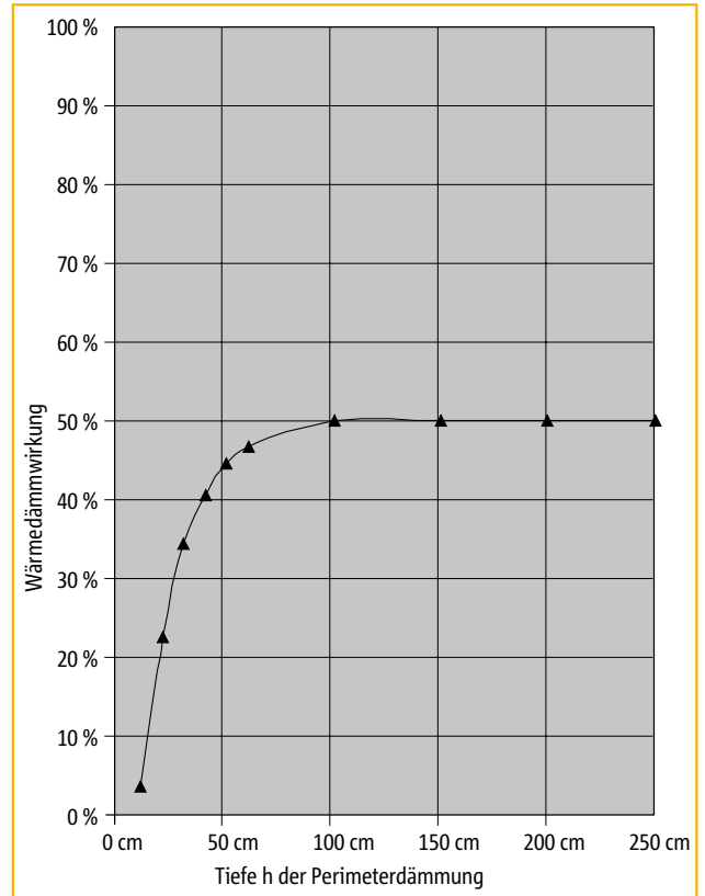
Abb. 5: Wärmedämmwirkung bei konstruktiver Dämmmaßnahme
