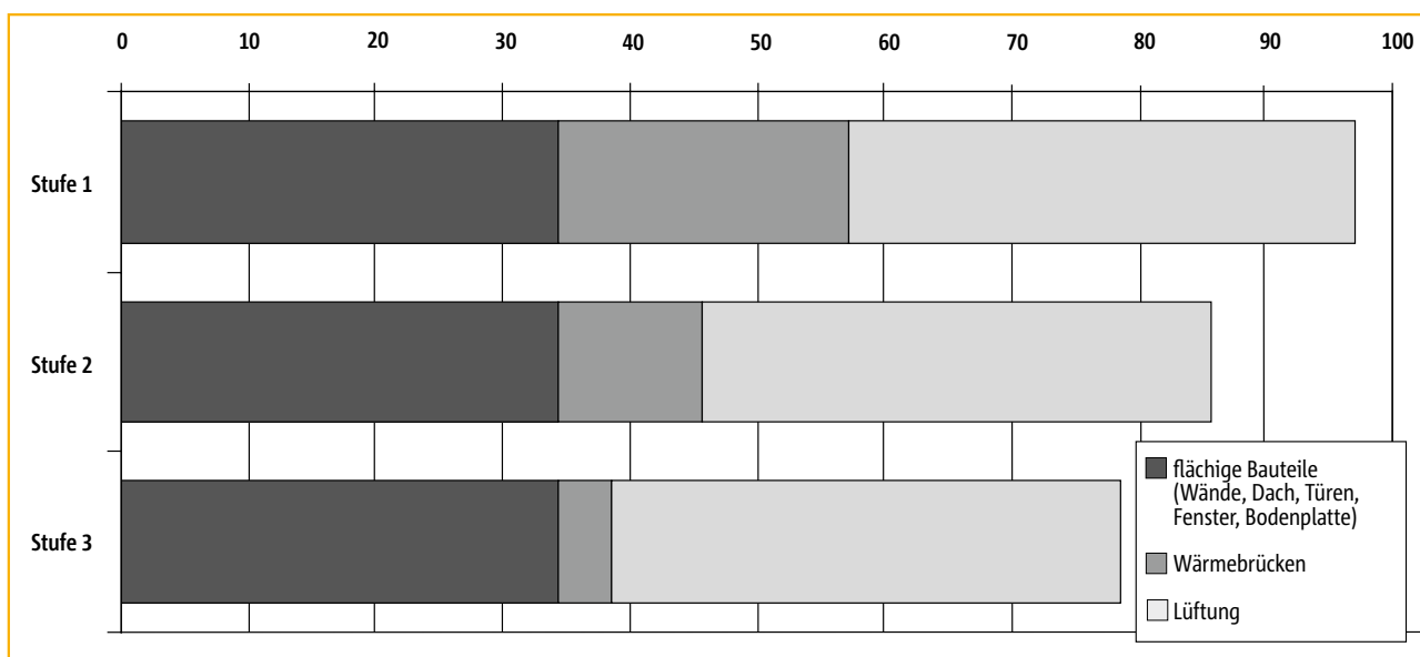
Diagramm 3: Auswirkungen des Wärmebrückeneinflusses auf die Heizenergiebilanz nach EnEV am Bsp. eines typischen Mehrfamilienhauses in Abhängigkeit von der Nachweis-Stufe (Quelle: „Bauphysik“, Heft 1, 02/2002)
