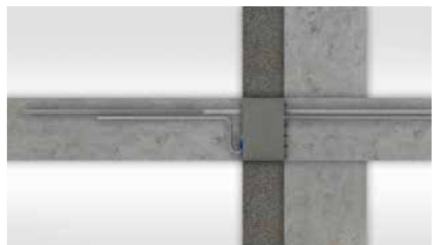
Frei auskragender Stahlbetonbalkon, nachträglich angeschlossen mit Schöck Isokorb® RT Typ K an bestehende Stahlbetondecke.
