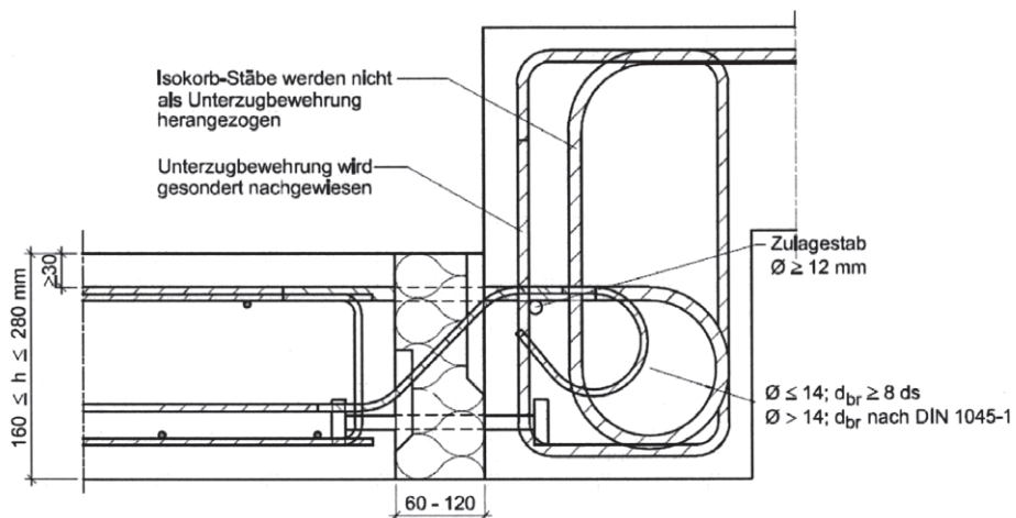
Abb. 15 Beispiel Schöck Isokorb Typ KX (Variante Höhenversatz) mit Aufhängebewehrung (balkenseitig)
