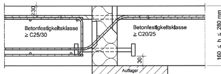
Abb. 11 Beispiel Schöck Isokorb Typ K mit Aufhängebewehrung nach Abschn. 3.2.1
