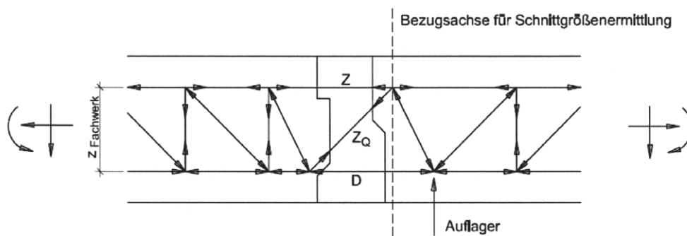
Abb. 30 Schöck Isokorb Typ K, Typ KF und Typ KX
