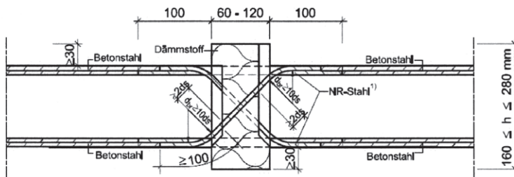
Abb. 17 Schöck Isokorb Typ D 1)
