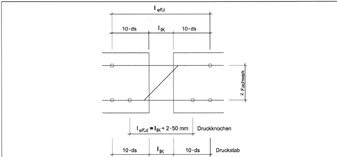
Abb. 38 l_{eff} für BS 500 NR, 1.4362 nach Datenblatt " Stahl mit Werkstoffnummer 1.4362 "
