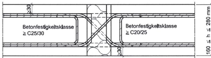
Abb. 18 Beispiel Schöck Isokorb Typ D mit Aufhängebewehrung nach Abschn. 3.2.1
