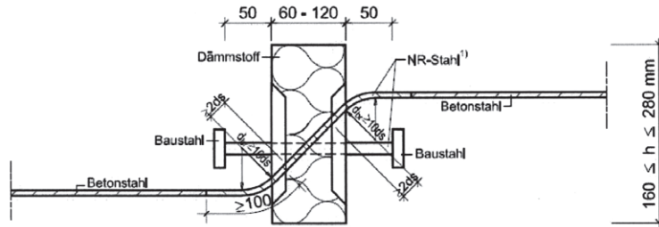
Abb.25 Schöck Isokorb Typ Q 1)
