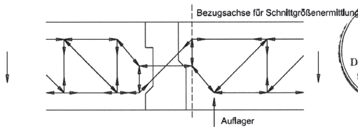
Abb. 35 Schöck Isokorb Typ Q
