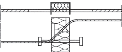
Abb. 2 Schöck Isokorb Typ KF
