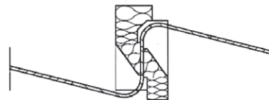
Abb. 6 Schöck Isokorb Typ V
