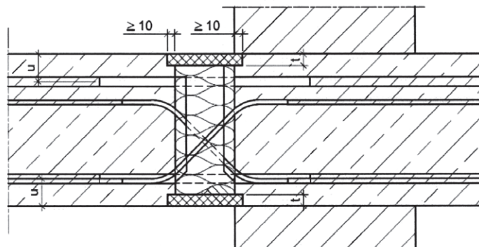
Abb. 41 Schöck Isokorb Typ D (F30/F90 bzw. R30/R90)
