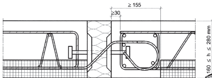
Abb. 48 Beispiel Schöck Isokorb Typ Q (mit abgelenktem Querkraftstab) mit Elementplatten
