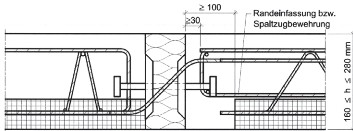
Abb. 47 Beispiel Schöck Isokorb Typ Q mit Elementplatten
