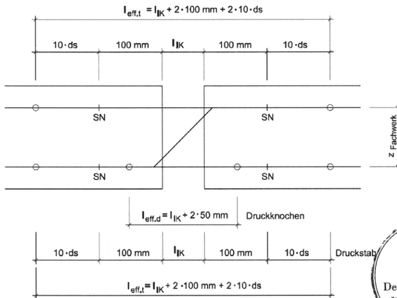
Abb. 39 l_{eff} für nichtrostenden glatten Stabstahl FkI, S 355 und S 460
