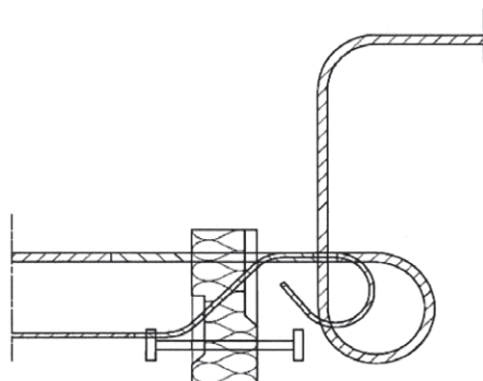
Abb. 4 Schöck Isokorb Typ KX
