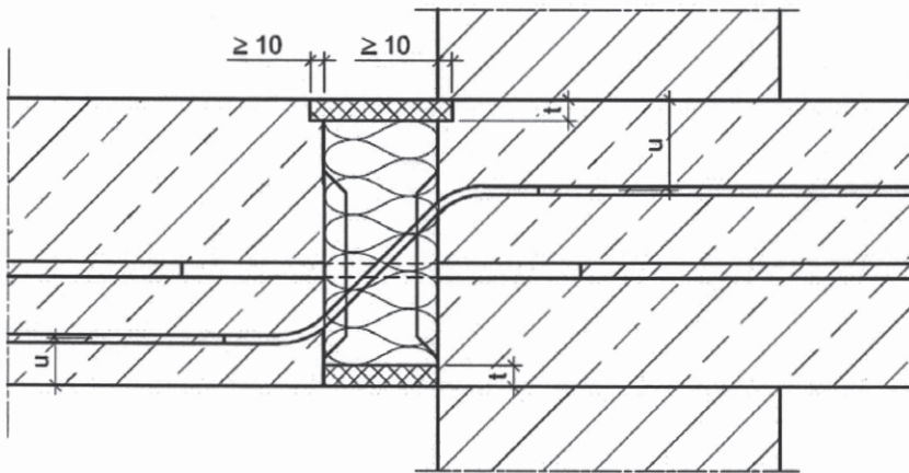
Abb. 43 Schöck Isokorb Typ Q und Typ QF (F30/F90 bzw. R30/R90)
