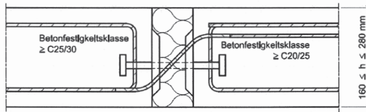
Abb. 26 Beispiel Schöck Isokorb Typ Q mit Aufhängebewehrung nach Abschn. 3.2.1
