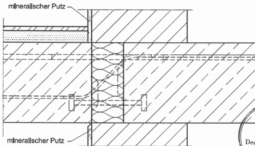
Abb. 44 Schöck Isokorb (F30 bzw. R30)
