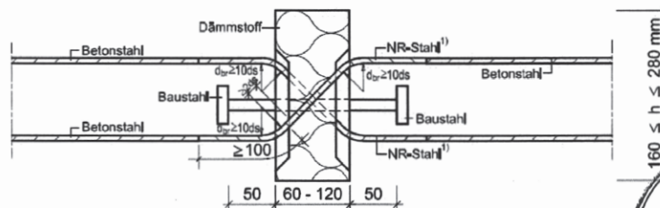
Abb. 27 Schöck Isokorb Typ Q+Q 1)
