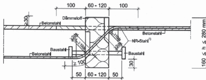
Abb. 9 Schöck Isokorb Typ K 1)
