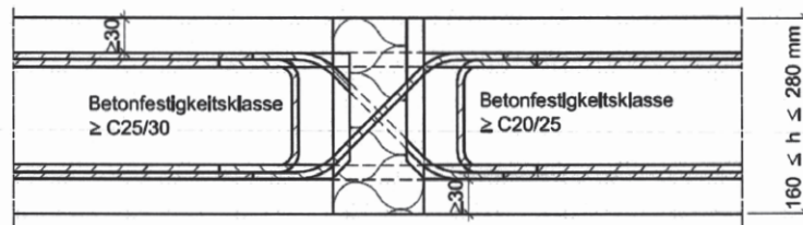
Abb. 18 Beispiel Schöck Isokorb Typ D mit Aufhängebewehrung nach Abschn. 3.2.1
