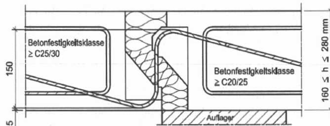
Abb. 23 Beispiel Schöck Isokorb Typ V mit Aufhängebewehrung nach Abschn. 3.2.1
