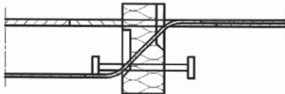
Abb. 1 Schöck Isokorb Typ K
