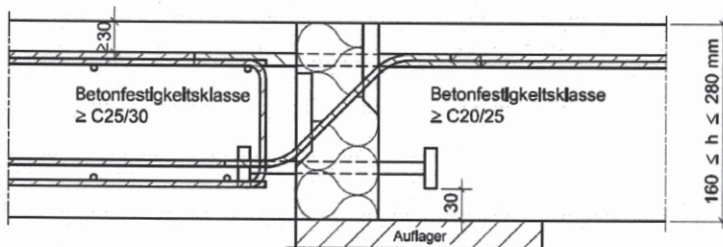
Abb. 11 Beispiel Schöck Isokorb Typ K mit Aufhängebewehrung nach Abschn. 3.2.1
