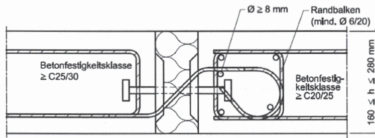
Abb. 29 Beispiel Schöck Isokorb Typ Q mit Aufhängebewehrung nach Abschn. 3.2.1 und Ausführung als Randbalken.
