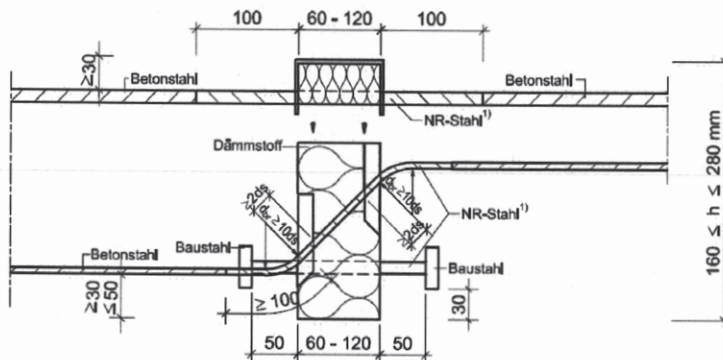
Abb. 10 Schöck Isokorb Typ KF 1)
