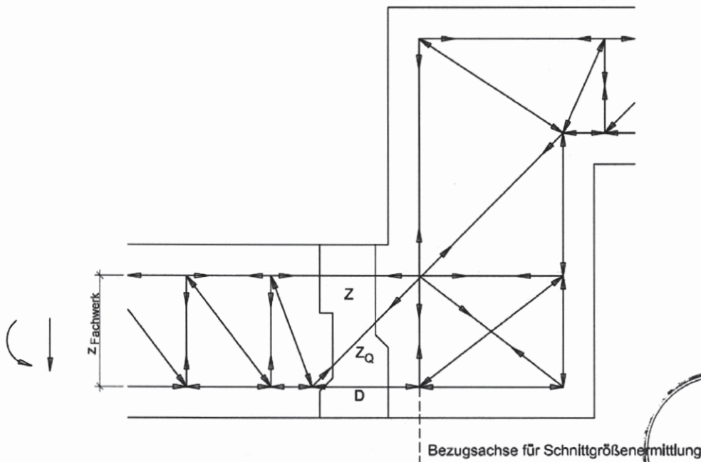
Abb. 31 Schöck Isokorb Typ K (Variante Höhenversatz)
