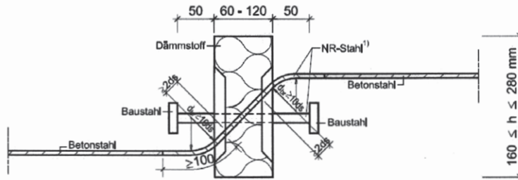
Abb.25 Schöck Isokorb Typ Q 1)
