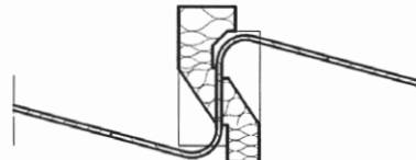
Abb. 6 Schöck Isokorb Typ V
