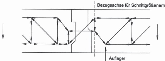
Abb. 35 Schöck Isokorb Typ Q
