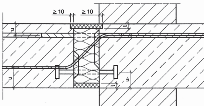
Abb. 40 Schöck Isokorb Typ KX, Typ K und Typ KF (F30/F90 bzw. R30/R90)
