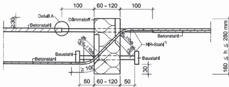
Abb. 12 Schöck Isokorb Typ K 1) mit Druck- Querkraft Kombination und abgestuften Nenndurchmesser der Zugstäbe
