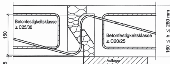
Abb. 20 Beispiel Schöck Isokorb Typ V mit Aufhängebewehrung nach Abschn. 3.2.1
