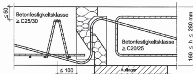
Abb. 21 Beispiel Schöck Isokorb Typ V mit Aufhängebewehrung nach Abschn. 3.2.1
