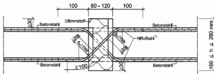
Abb. 17 Schöck Isokorb Typ D 1)
