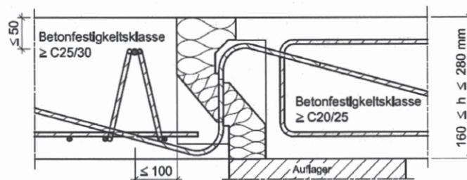
Abb. 24 Beispiel Schöck Isokorb Typ V mit Aufhängebewehrung nach Abschn. 3.2.1
