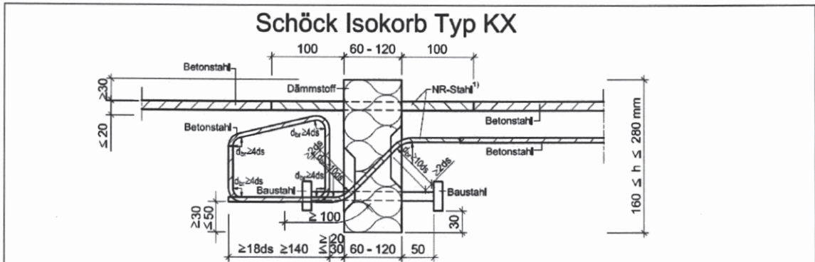
Abb. 14 Schöck Isokorb Typ KX 1) mit Druck- Querkraft Kombination und integrierter Aufhängebewehrung.
