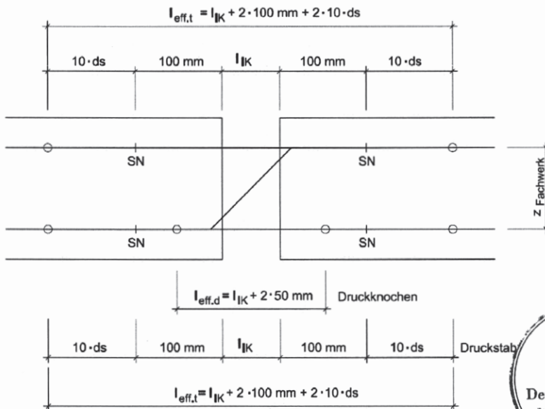
Abb. 39 l_{eff} für nichtrostenden glatten Stabstahl Fkl. S 355 und S 460
