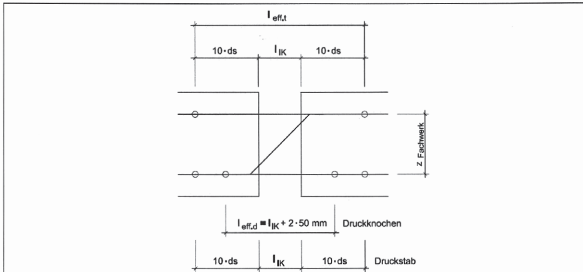
Abb. 38 l_{eff} für BSt 500 NR, 1.4362 nach Datenblatt " Stahl mit Werkstoffnummer 1.4362 "
