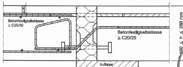
Abb. 16 Beispiel Schöck Isokorb Typ KX mit integrierter Aufhängebewehrung
