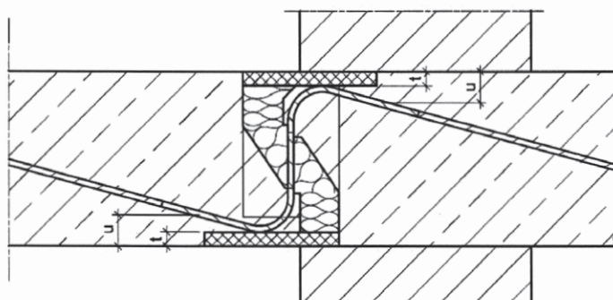
Abb. 42 Schöck Isokorb Typ V (F30/F90 bzw. R30/R90)
