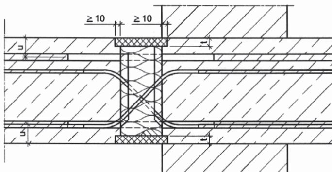
Abb. 41 Schöck Isokorb Typ D (F30/F90 bzw. R30/R90)
