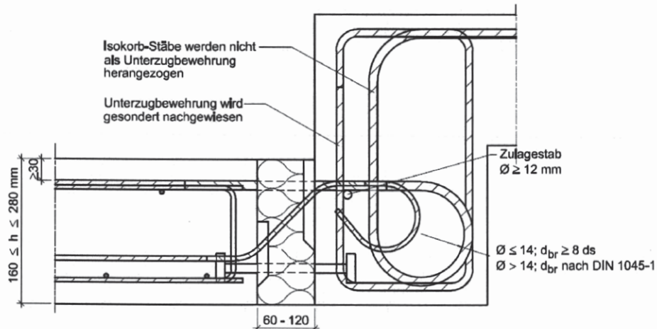
Abb. 15 Beispiel Schöck Isokorb Typ KX (Variante Höhenversatz) mit Aufhängebewehrung (balkonseitig)
